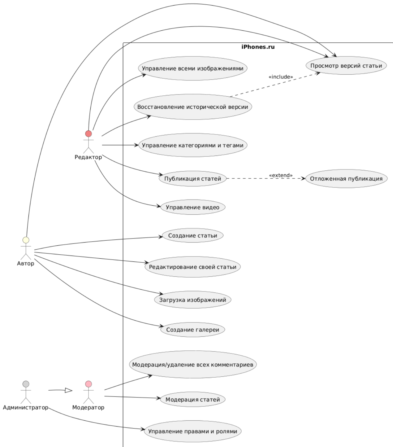
Рис. 1: UseCase1
