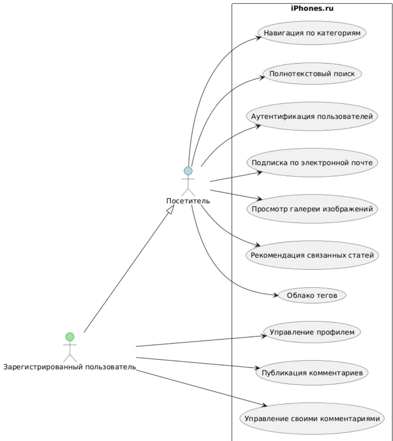
Рис. 2: UseCase 2
